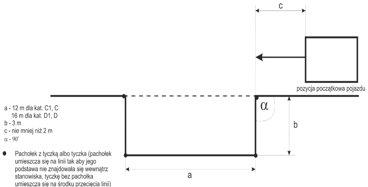
Rysunek nr 4. Parkowanie równoległe (wjazd tyłem - wyjazd przodem).
