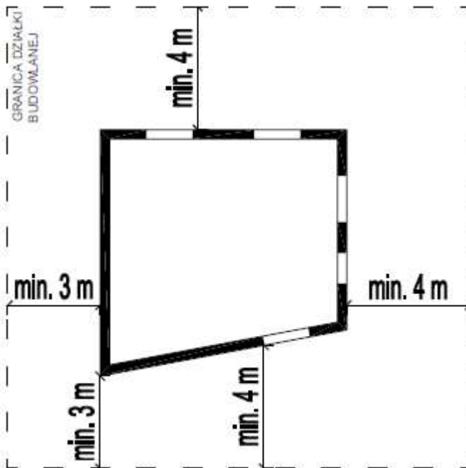
Rys. 6 Budynek ze ścianą usytuowaną w sposób inny niż równoległy w stronę granicy działki budowlanej – § 12 ust. 3a.
