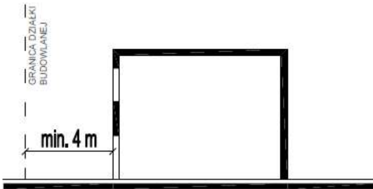
Rys. 2 Budynek zwrócony ścianą z oknami lub drzwiami w stronę granicy działki budowlanej – § 12 ust. 1 pkt 1.
