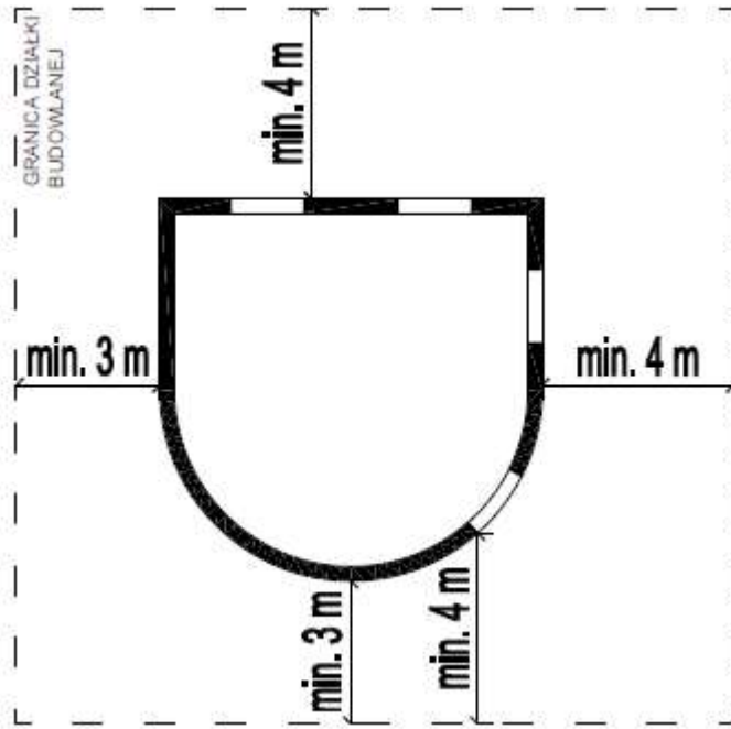
Rys. 7 Budynek ze ścianą usytuowaną w sposób inny niż równoległy w stronę granicy działki – § 12 ust. 3a.
